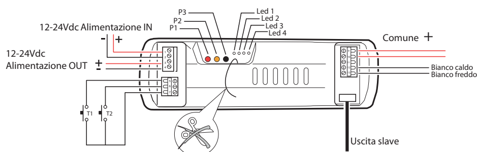
Schema di collegamento
