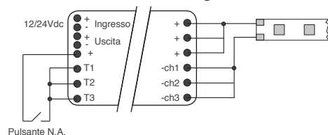
Schema di collegamento 1
