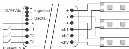
Schema di collegamento 2
