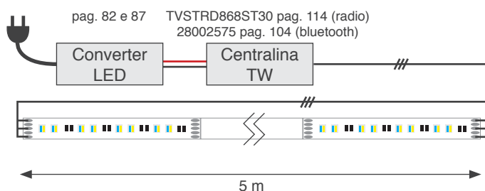
Alimentazione dalle estremità
