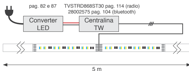
Alimentazione in centro
