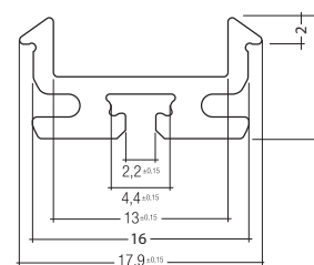
Dimensioni in mm
